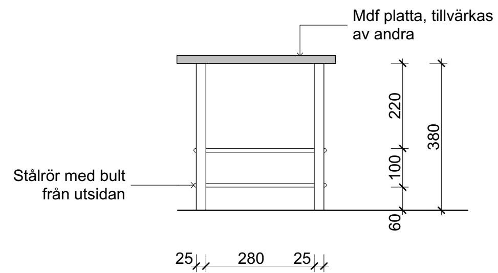
SIDOVY Skala 1:10
