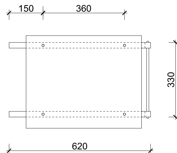
PLAN Skala 1:10
